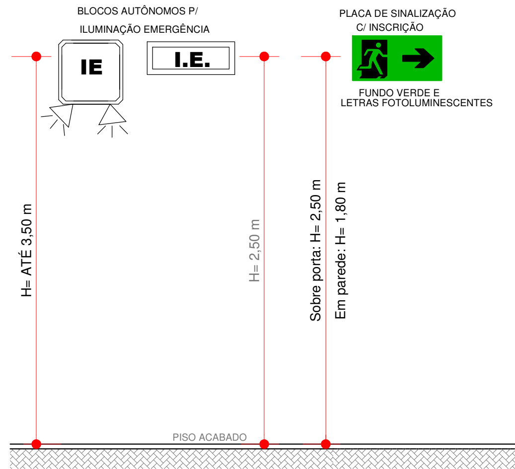
ALTURA DAS LUMINÁRIAS E SINALIZAÇÕES SEM ESCALA
