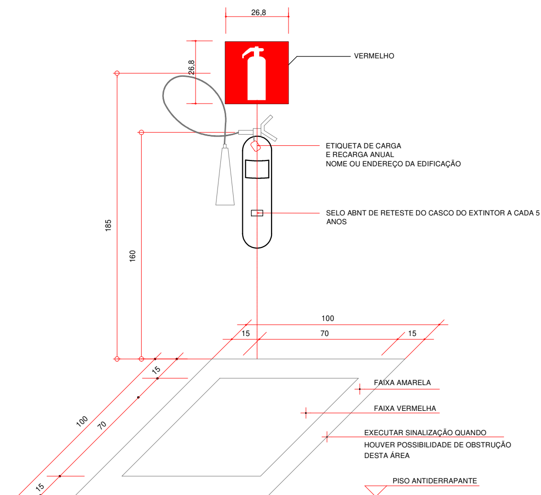
EXTINTOR SEM ESCALA
